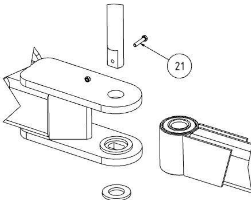
Rys.11 : Łączenie ramion wysięgnikowych
