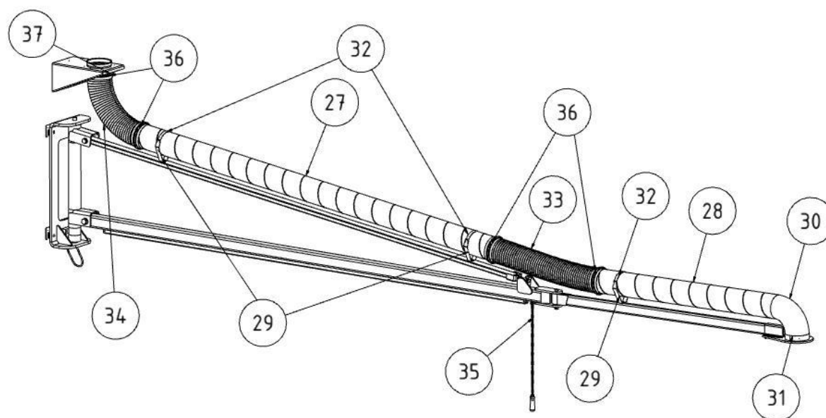
Rys.14 : Montaż rury falistej
