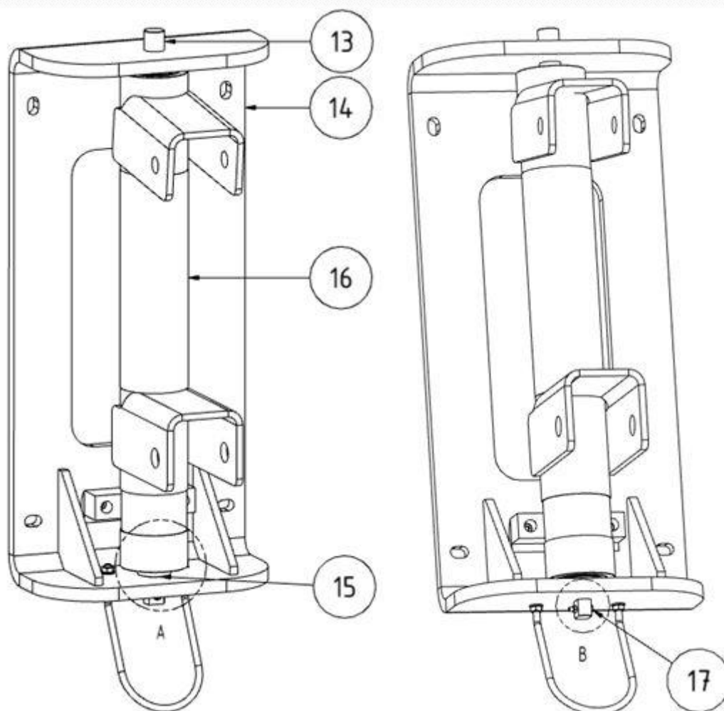
Rys.6 : Uchwyt ramienia wysięgnikowego
