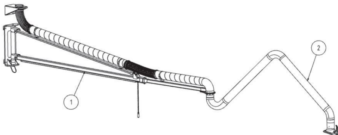
Rys. 1: Ramię odciągowe z ramieniem wsięgnika wychylnego
