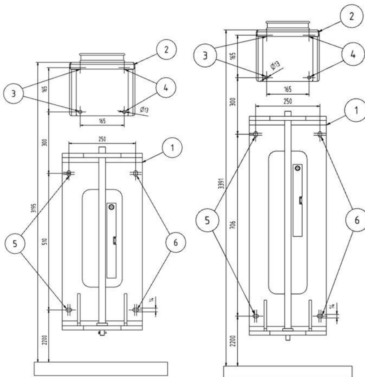
Rys.5 : Uchwyt ścienny
