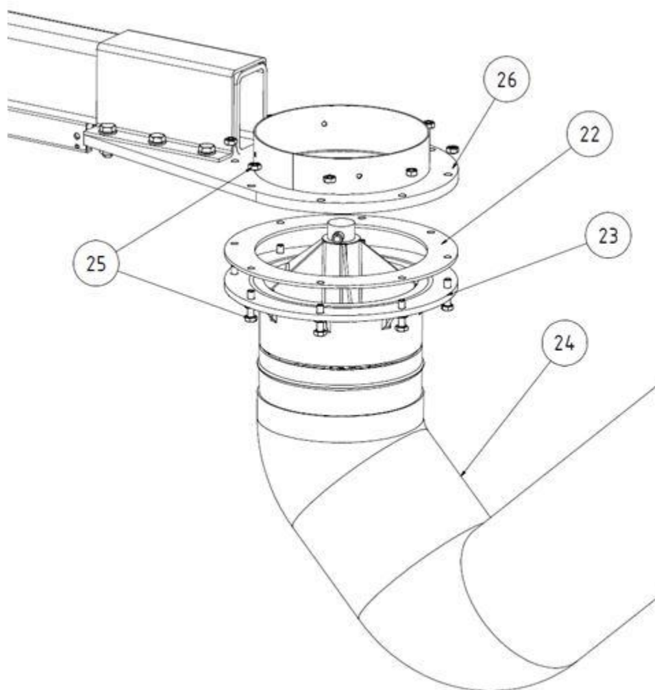
Rys.12 : Ramię odciągowe na ramieniu wysięgnika
