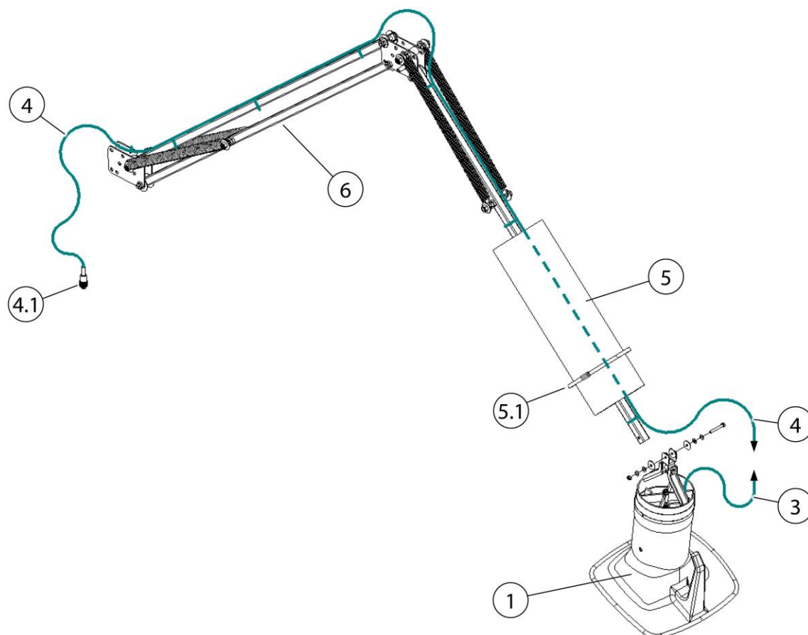
Rys.18 : Układanie kabli – ramię odciągowe 2–4 metry
